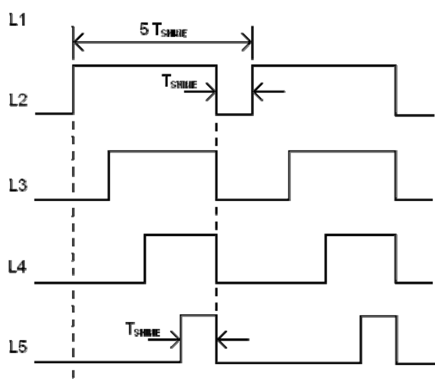
图5 一级电量 L1~L5 端口波形图
