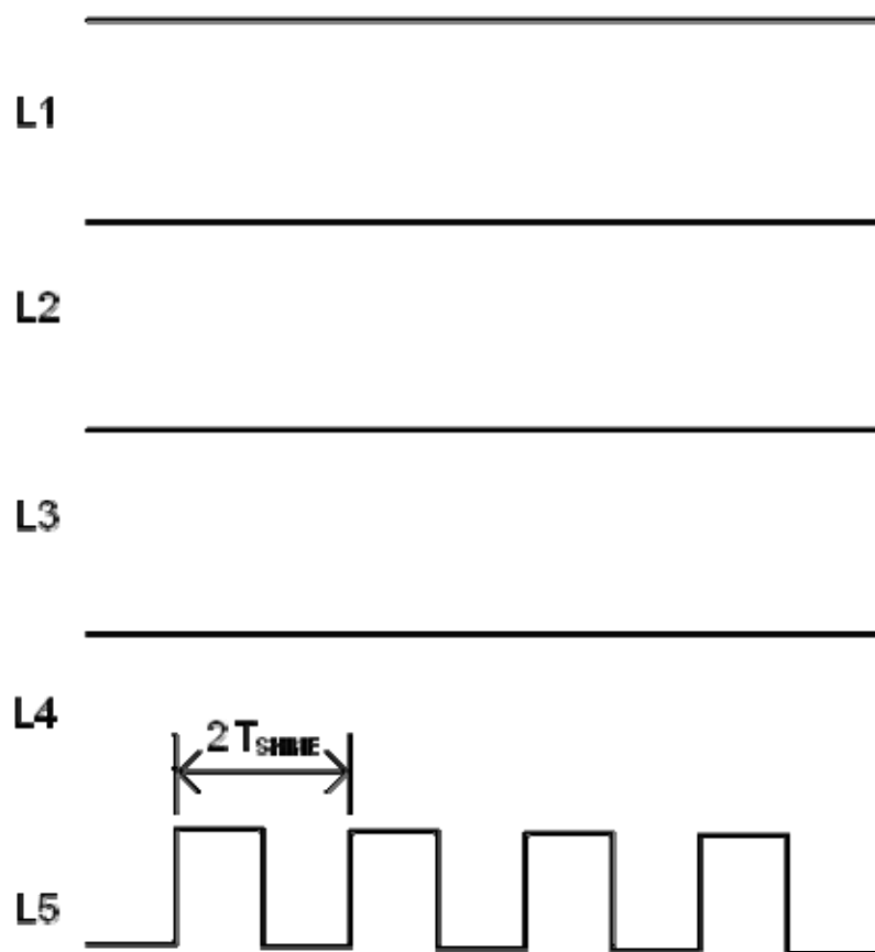
图 8 四级电量 L1~L5 端口波形图
